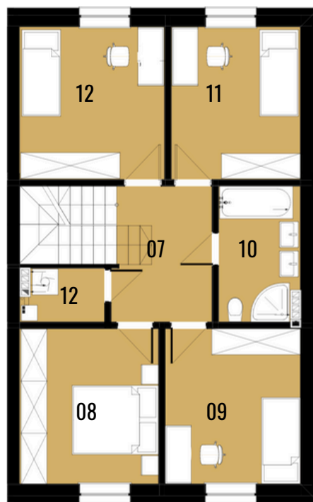
RZUT PIĘTRA
